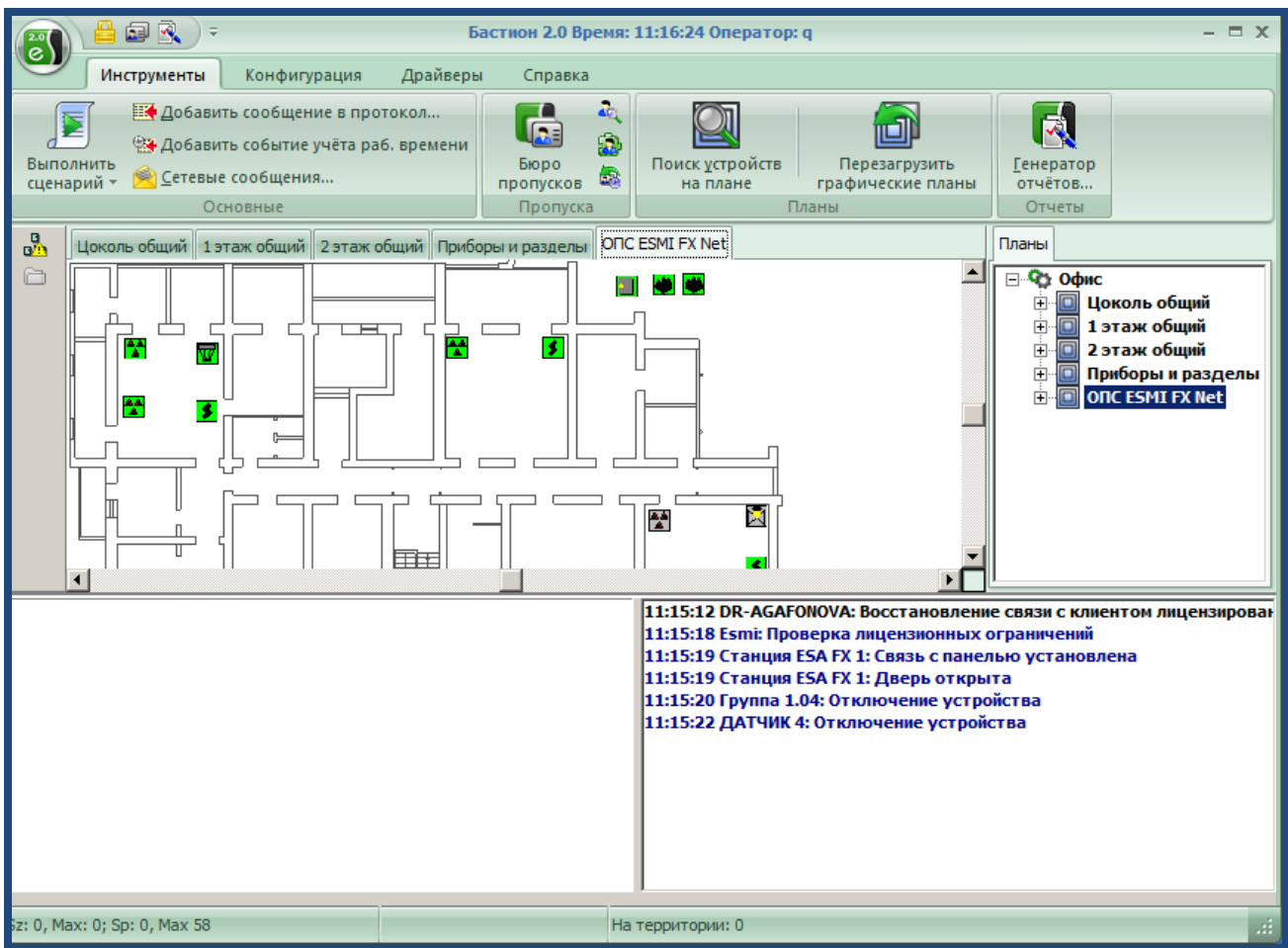
Рисунок 5 – Сообщения получения текущего состояния устройств
