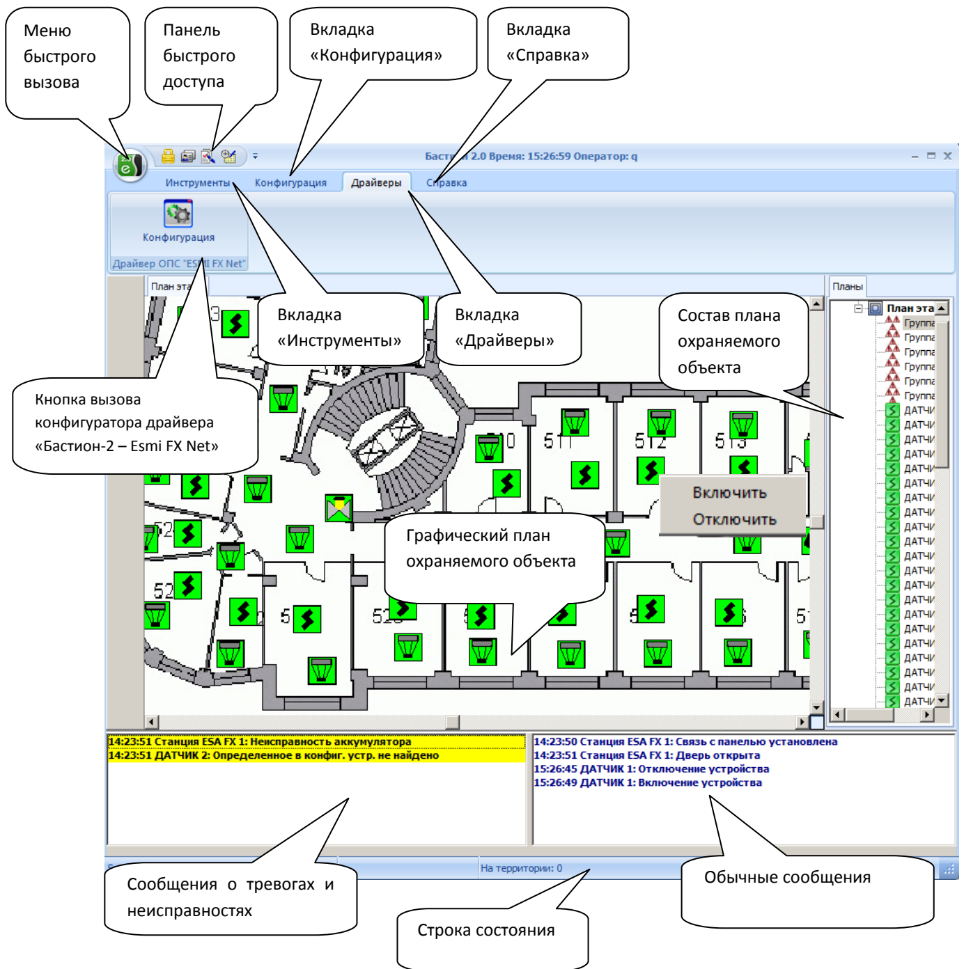
Рисунок 1 – Главное окно «Бастион-2» с установленным драйвером «Бастион-2 – Esmi FX Net»
