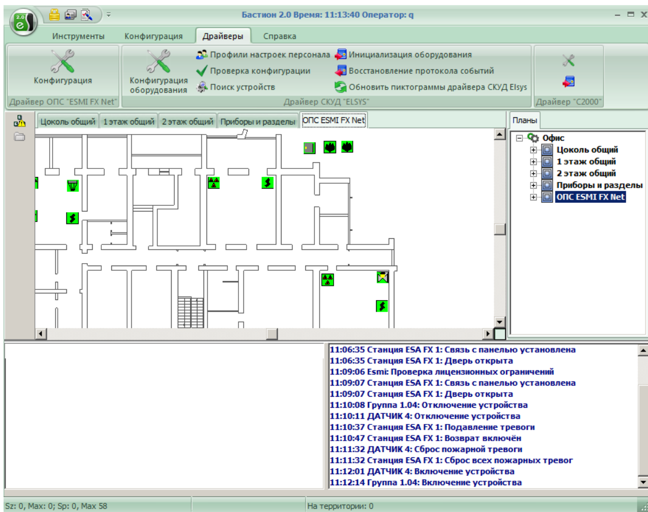
Рисунок 4 – Сообщения, связанные с управлением устройствами
