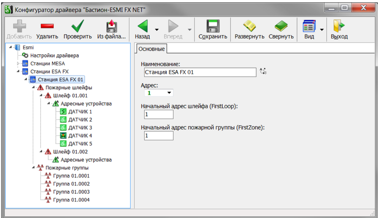
Рисунок 21 Конфигурация станции из файла
