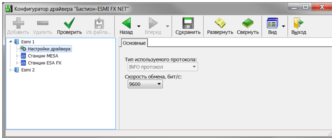
Рисунок 28 Настройки драйвера
