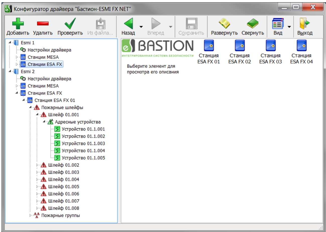
Рисунок 23 Пользовательский интерфейс configurатора
