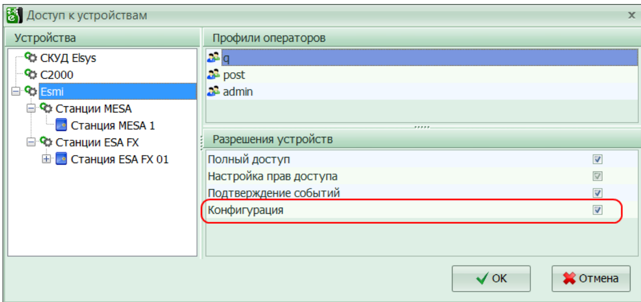
Рисунок 22 Разрешение на работу в конфигураторе драйвера «Бастион-2 – Esmi FX Net»
