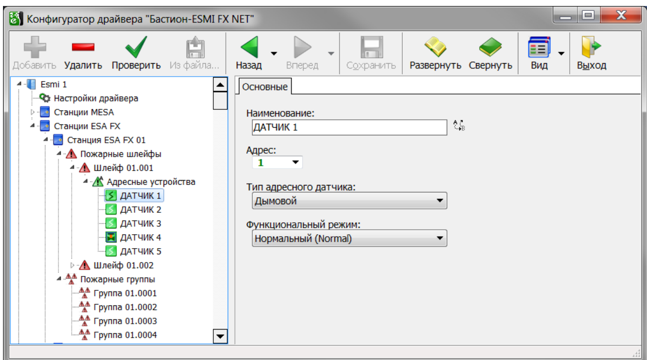
Рисунок 37 - Свойства адресного датчика
