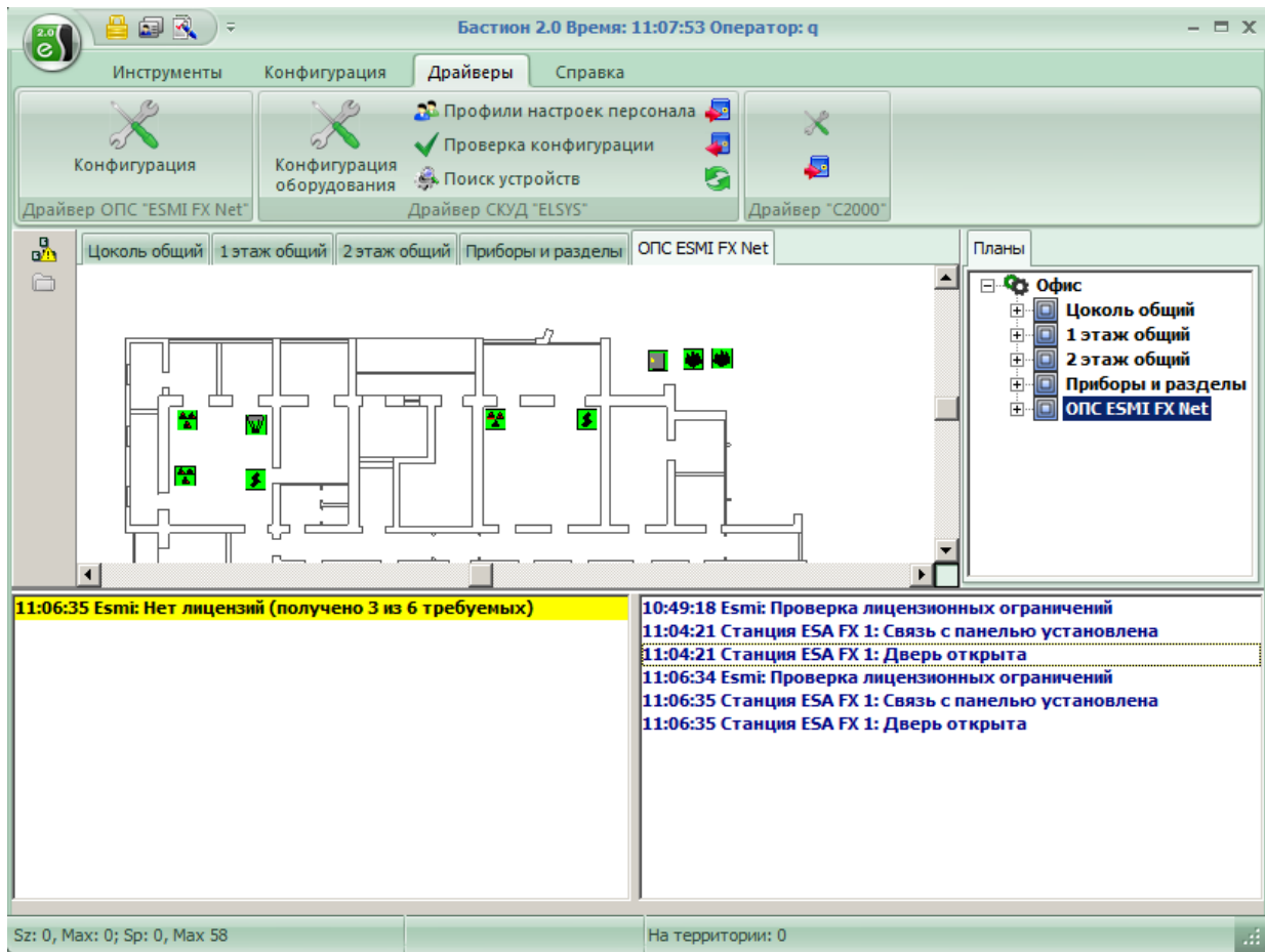
Рисунок 2 – Сообщения при загрузке «Бастион-2»
