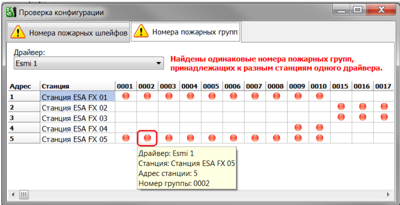
Рисунок 40 - Результаты проверки уникальности номеров пожарных групп при наличии ошибок
