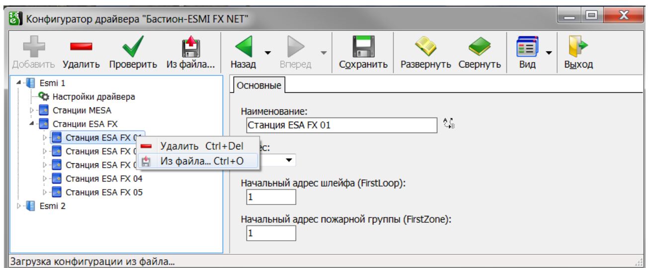
Рисунок 31 - Чтение конфигурации станции ESA FX из файла
