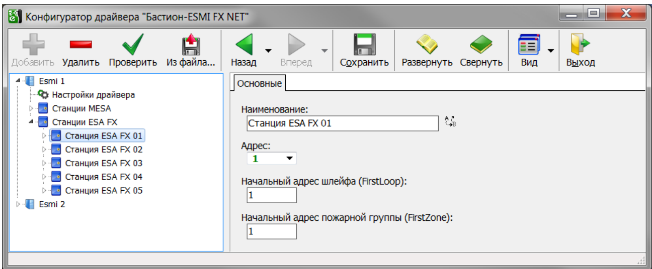
Рисунок 30 - Свойства станции ESA FX
